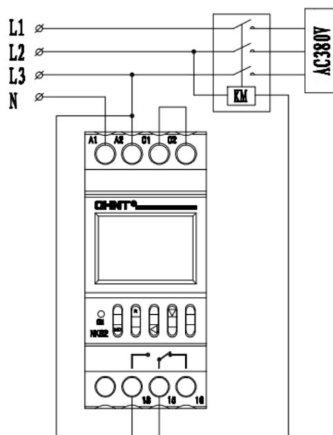
Figura 5 - Conexión trifásica con bobina de de contactor a 380Vca (Ie: 1.5A [KM])
