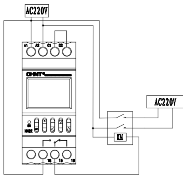
Fig. 3 - Conexión expandida monofásica(NXJ-A/NXC-6)
