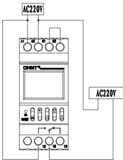
Figura 2 - Conexión directa monofásica
