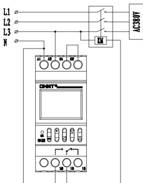
Figura 4 - Conexión trifásica con bobina contactor a 220Vca (Ie: 3A [KM])
